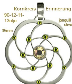
90-12-27 Erinnerung 13 Kristalle
